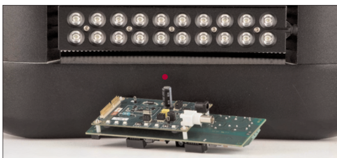
Applicazione per Street Lighting da 50 W dotata di sistema di controllo remoto
